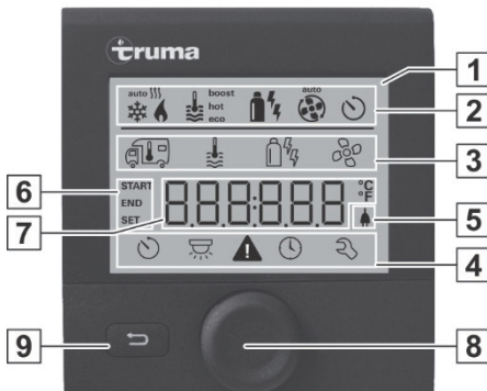
Kuva 140: Digitaalinen TRUMA-käyttölaite CP Plus
