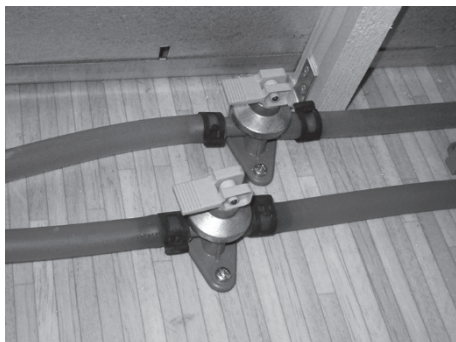
Kuva 178: Tyhjennysventtiilit suljettu
