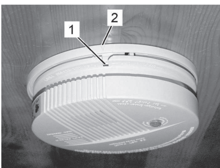
Kuva 229: Rungon kiinnitys paikoilleen
