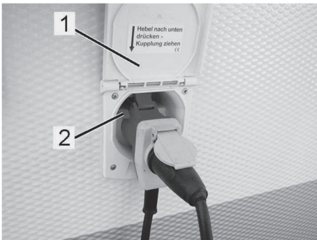
Kuva 59: Verkkoliitäntä
