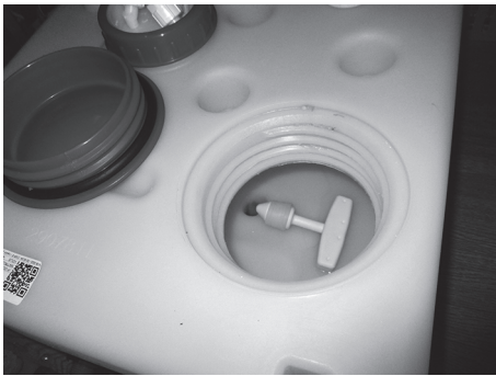
Kuva 109: Tyhjennystulppa raikasvesisäiliössä
