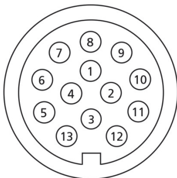
Kuva 2: 13-napainen pistoke
