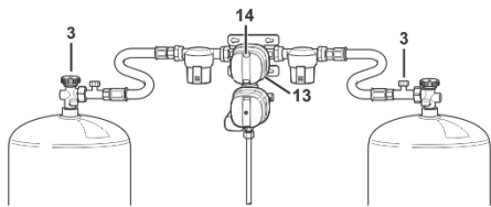
Kuva 117: Kaasupaineensäädinsarja
