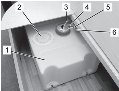
Kuva 96: Raikasvesisäiliö, esimerkki
