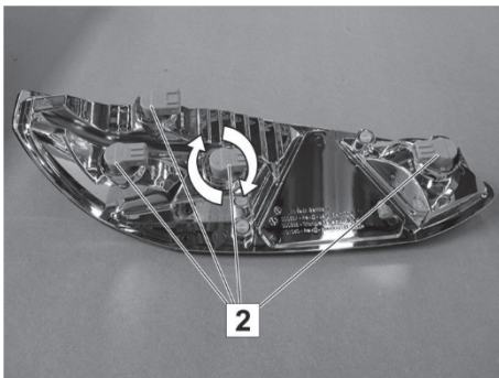
Kuva 225: Takavalo (takapuoli)
