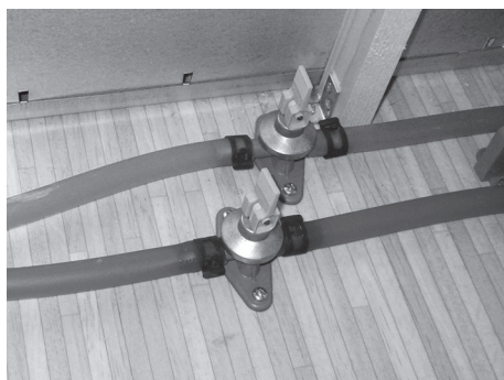
Kuva 104: Tyhjennysventtiili auki
