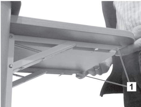
Kuva 208: Kääntökonsolin lukituksen vapauttaminen
