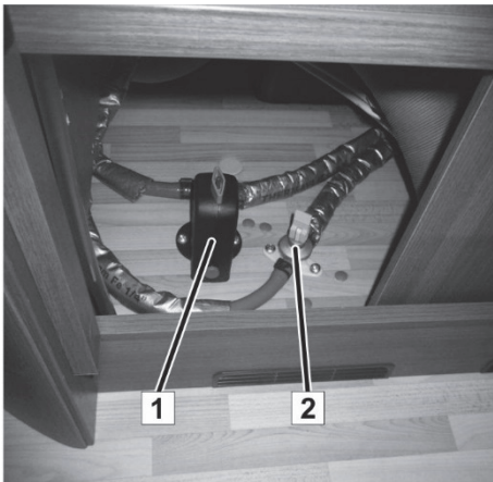
Kuva 110: Truma-Combi-lämmityslaitteen tyhjennysventtiilit
