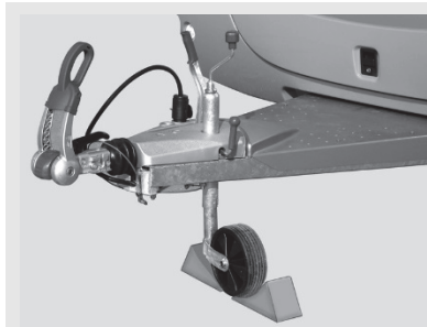
Kuva 218: Tukipyörän varmistaminen
