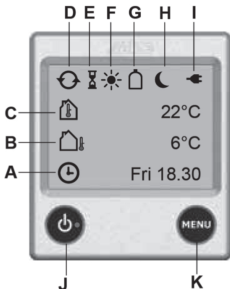
Kuva 162: Käyttöelementit
