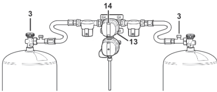
Kuva 120: Kaasupaineensäädinsarja
