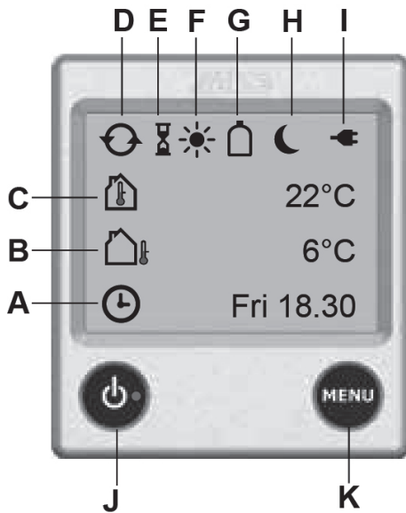
Kuva 88: Käyttöelementit
