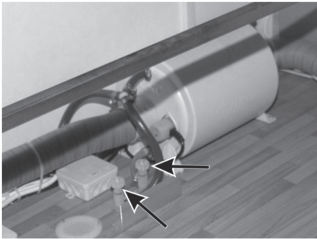
Kuva 101: TRUMA-lämmityssäiliö ja vedentyhjennysventtiilit
