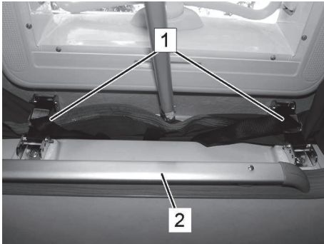
Kuva 192: Nostokaton kääntäminen auki
