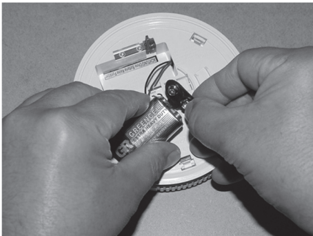
Kuva 228: Nepparipariston vaihto
